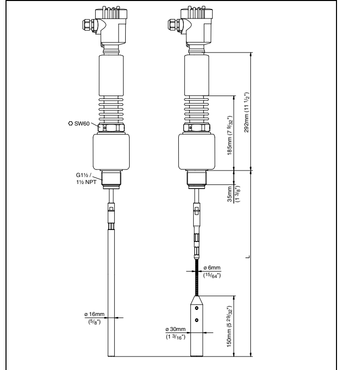
Fig. 30: VEGAFLEX 66 - cable, rod version (-200 ... +400 °C/-328 ... +752 °F)
